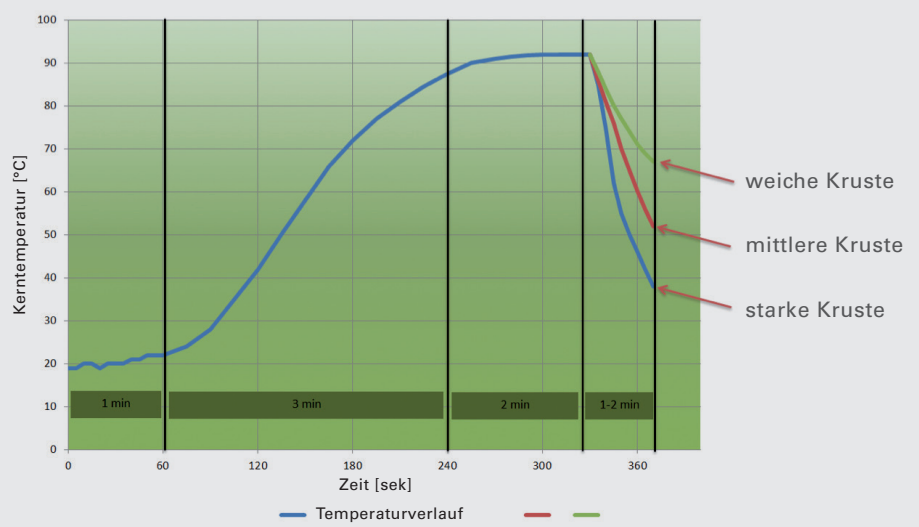
Kerntemperaturverlauf beim Vakuumbackprozess
